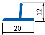
Art. Nr.: 1107 T-Schiene
