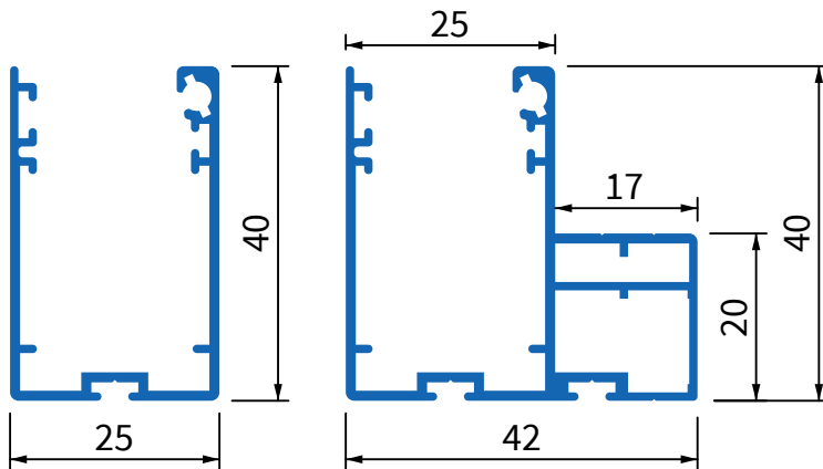
2305 Rollo Führungsschiene, schmal
