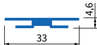
1709 Lichtschachtprofil, abgerundet mit Fahne
