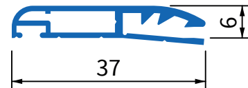
1707 Lichtschachtprofil, abgerundet
