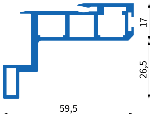
1730 Gittersafeprofil
