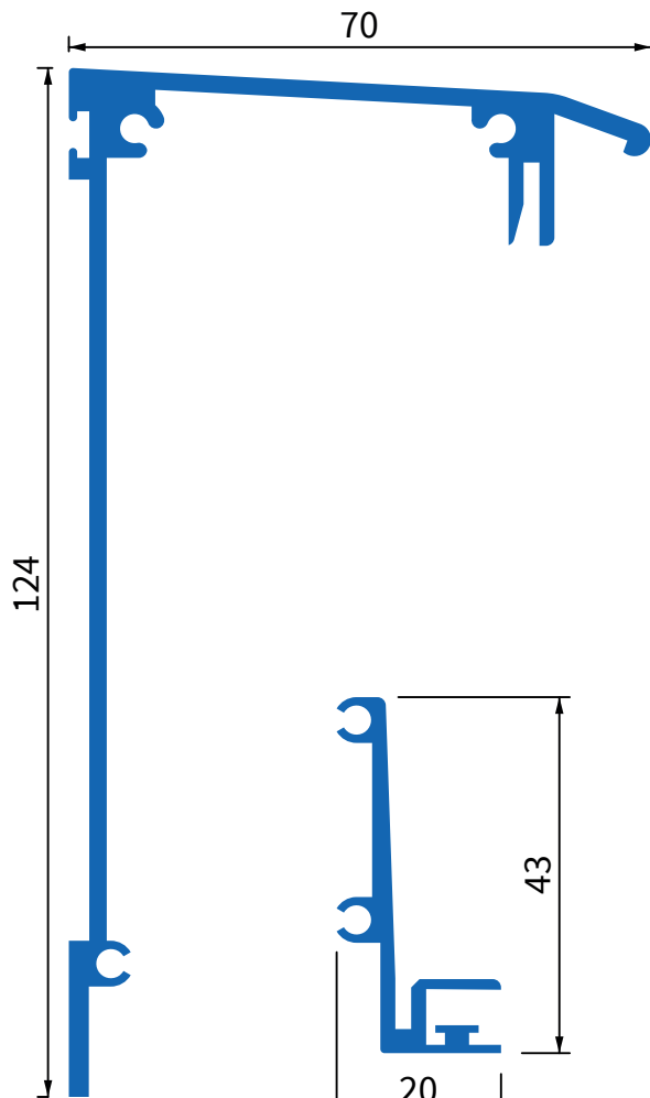
1736 Lüftungsprofil
