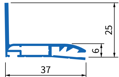
1708 Lichtschachtprofil, abgerundet mit Randbürstenaufnahme
