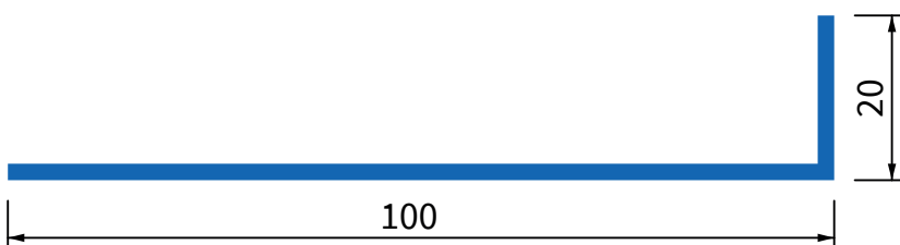
1610 L-Winkelprofil 100 x 20 x 2 mm*
